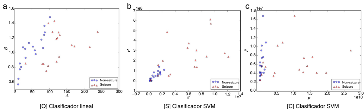
Figura 1 – Diagrama de dispersión de la banda delta. a) [Q] escala A eje- x y forma B eje- y . b) [S] energía \varepsilon eje- x y potencia P eje- y . c) [C] frecuencia F eje- x y potencia P eje- y . Todos los métodos permiten una discriminación entre eventos de no-crisis (círculos azules, non-seizure ) y eventos de crisis (triángulos rojos, seizure ). En la edición online podrá consultar los colores de las figuras.
