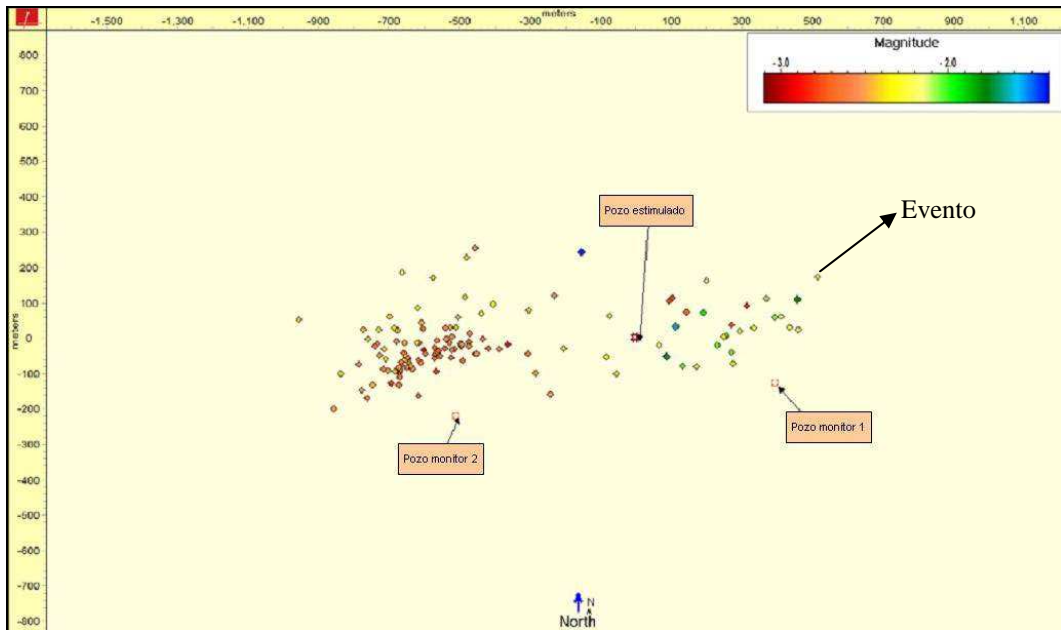
Figura 17. Esquema en planta de ubicación no simétrica de pozos y geófonos en la operación. La magnitud y ubicación del evento microsísmico y la geometría de la fractura dependerán de la posición relativa de pozos monitores y pozo estimulado.
