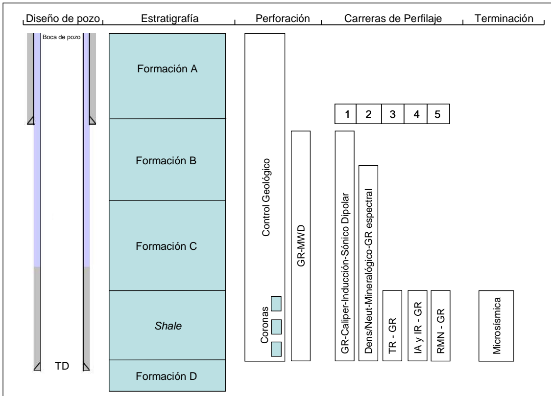
Figura 20. Esquema de adquisición de información y toma de muestras en una etapa exploratoria para un pozo con objetivo no convencional. TR: Testigos Laterales Rotados; IA: Imagen Acústica; IR: Imagen Resistiva.
