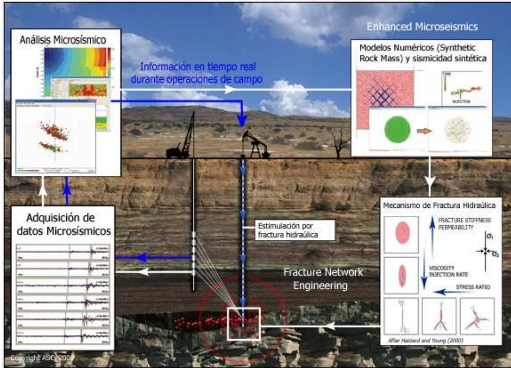
Figura 15. Esquema de la operación de campo.
