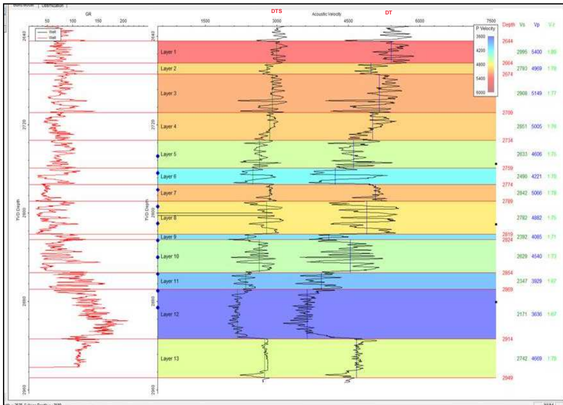
Figura 16. Ejemplo de modelo de velocidades intervalarias determinado in situ .
