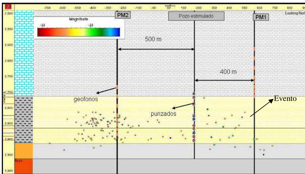
Figura 18. Esquema de detección de eventos en perfil, en el caso más genérico, donde no hay simetrías respecto del pozo fracturado de la ubicación de la ristra de geófonos.
