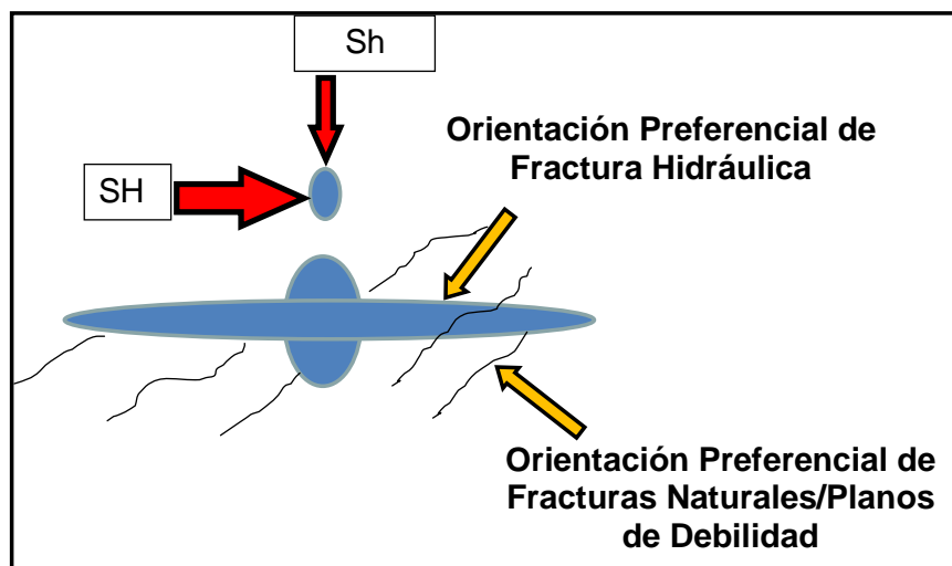
Figura 19. Esquema de sistemas de fracturas.
