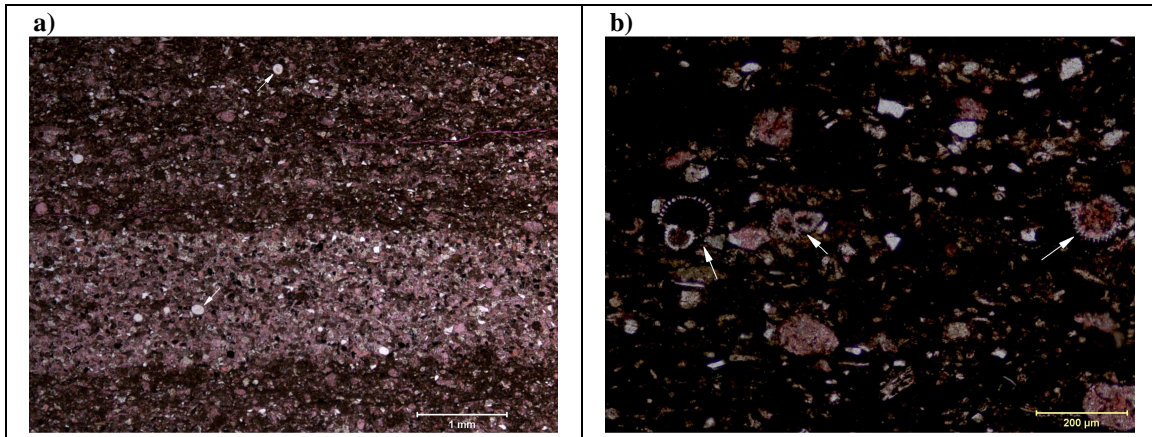
Figura 11. Ejemplos de cortes delgados. a) Laminación bien definida en un mudstone calcáreo, b) Fósiles (radiolarios) reemplazados por cuarzo microcristalino.
