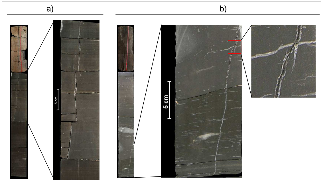
Figura 12. Fotografías de coronas con fracturas generadas durante la expulsión del hidrocarburo. a) Intensa laminación en el 2/3 inferior de la corona. Fracturas naturales subverticales y subparalelas de hasta 1 mm de ancho rellenas parcial o totalmente con calcita, yeso, pirita y bitumen. b) fractura subvertical de 1,6 mm de ancho con poros de hasta 0,3 mm de diámetro.
