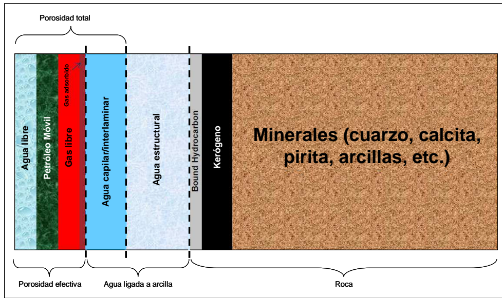
Figura 8. Fluidos y porosidades presentes en un shale .
