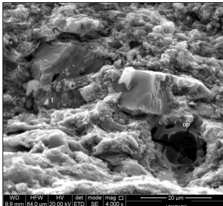
Figura 10. Ejemplo de imagen obtenida a partir del SEM. (Op: partícula orgánica, f: fósil calcáreo).
