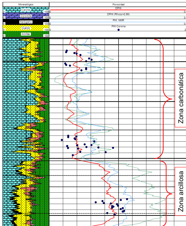
Figura 6. Comparación entre porosidades totales obtenidas a partir del perfil de densidad con densidad de grano constante (verde), con densidad de grano variable (rojo) y del perfil de resonancia (azul). Los datos de laboratorio se presentan como círculos azules.
