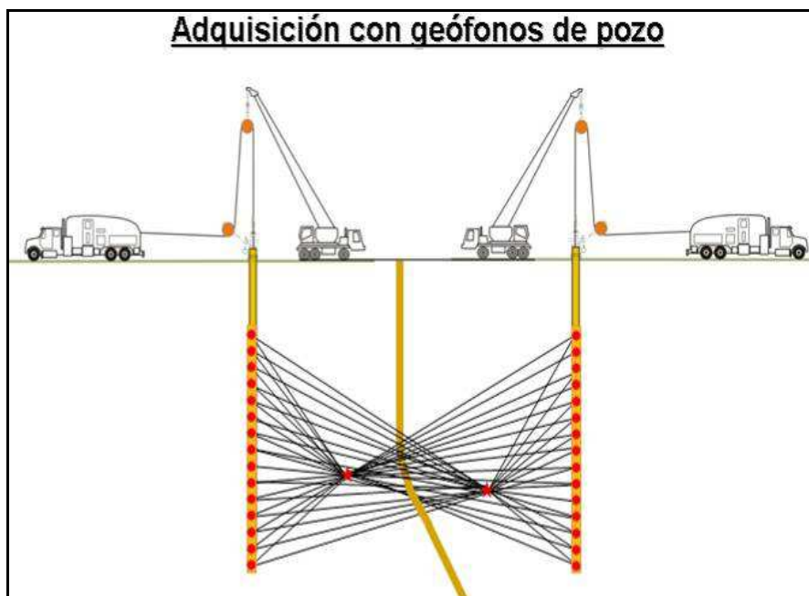
Figura 14. Esquema de la puesta en estación. Se pueden apreciar dos pozos monitores con la ristra de geófonos en su interior y en el centro, el pozo desviado donde se realizará la fractura hidráulica.
