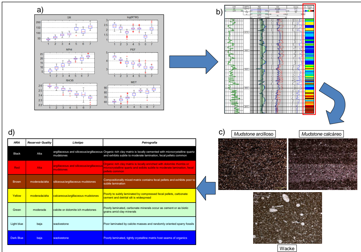
Figura 7. Flujo para la determinación de litofacies a partir de métodos estadísticos aplicados a perfilajes eléctricos disponibles. a) Determinación de electro-facies; b) presentación del perfil de facies; c) descripción petrográfica de muestras de distintas clases; d) determinación de litofacies.
