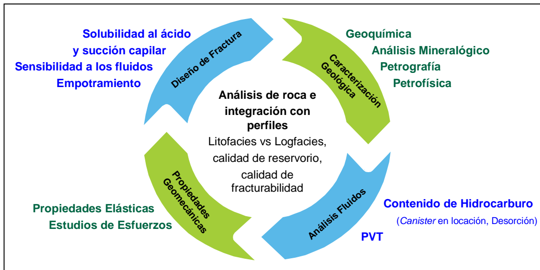
Figura 4. Diagrama de flujo generalizado para la caracterización del reservorio, optimización de la estimulación, determinación de la productividad y planificación del desarrollo.
