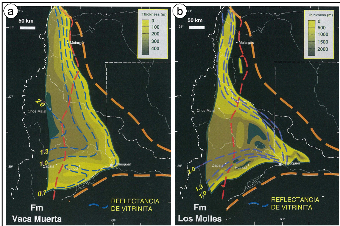
Figura 3. Mapa de reflectancia e isopáquico de las formaciones a) Vaca Muerta y b) Los Molles. Trazo rojo: faja plegada, trazo naranja: límite de cuenca (Legarreta et al. 2005).
