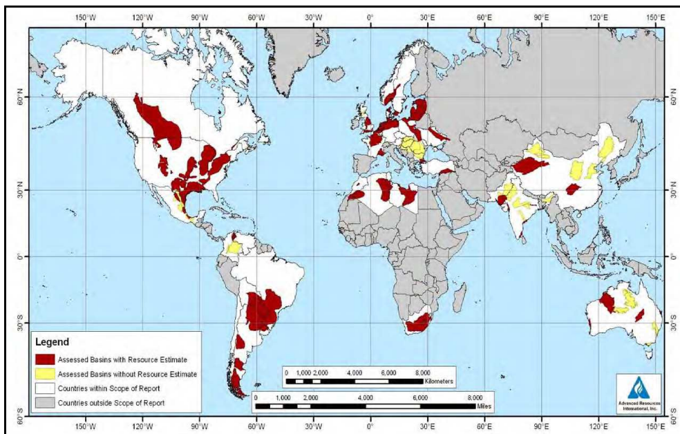
Figura 1. Cuencas de shale estudiadas alrededor del mundo (EIA, 2011).
